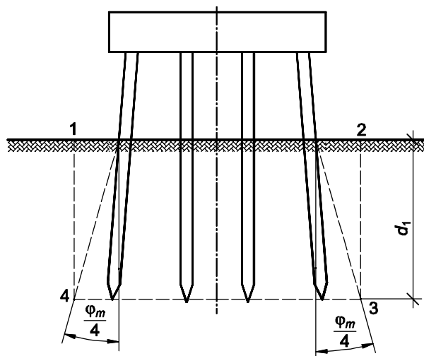
Рисунок Л.3 — Условный свайный фундамент с ростверком, расположенным над грунтом, при угле наклона свай менее \varphi_m/4
