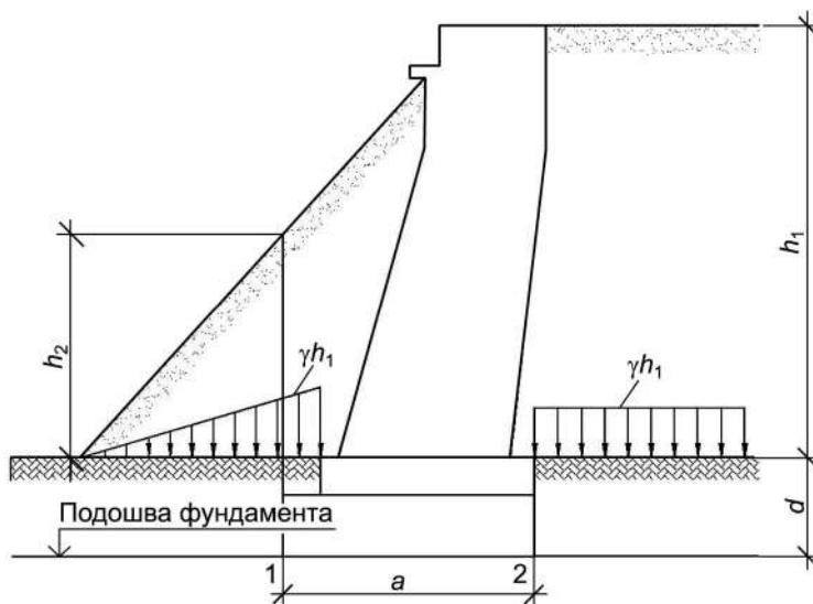
Рисунок М.1 — Схема распределения дополнительного давления от веса подходной насыпи на грунты основания обсыпного устоя
