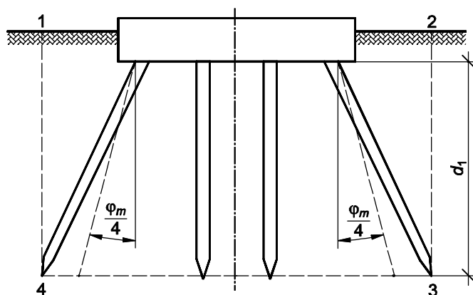
Рисунок Л.2 — Условный свайный фундамент с ростверком, заглубленным в грунт, при угле наклона свай более \varphi_m/4
