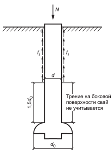
Рисунок 7.1 — Схема к расчету сопротивления на боковой поверхности ствола сваи с уширением в песчаном грунте
