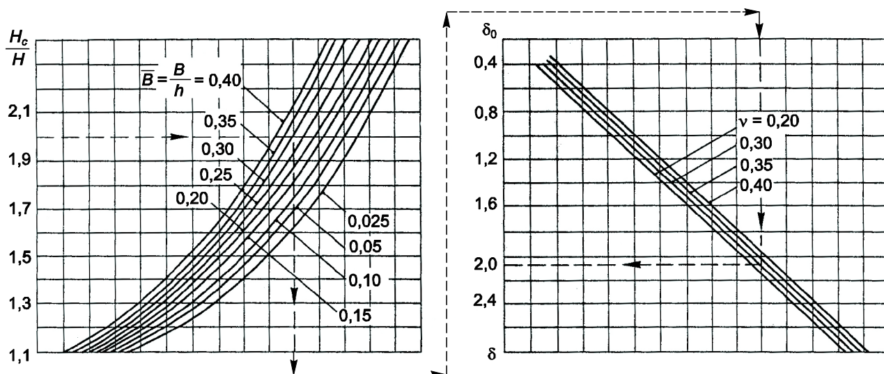
Рисунок В.1 — Номограмма для определения значений \delta_0
