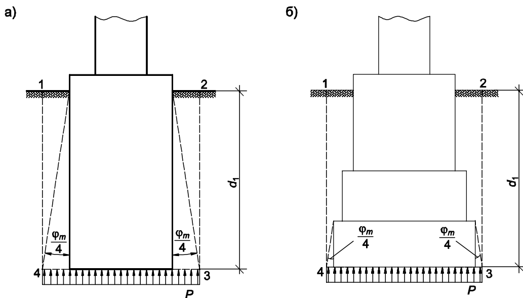
Рисунок Л.5 — Условный фундамент из опускающего колодца: а — без уступов; б — с уступами
