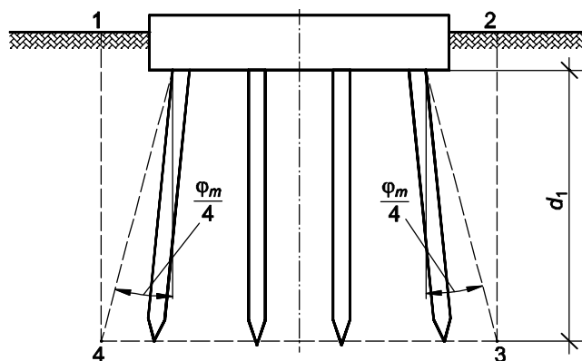
Рисунок Л.1 — Условный свайный фундамент с ростверком, заглубленным в грунт, при угле наклона свай менее \varphi_m/4
