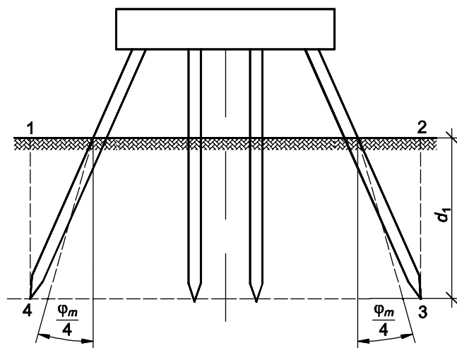
Рисунок Л.4 — Условный свайный фундамент с ростверком, расположенным над грунтом, при угле наклона свай более \varphi_m/4
